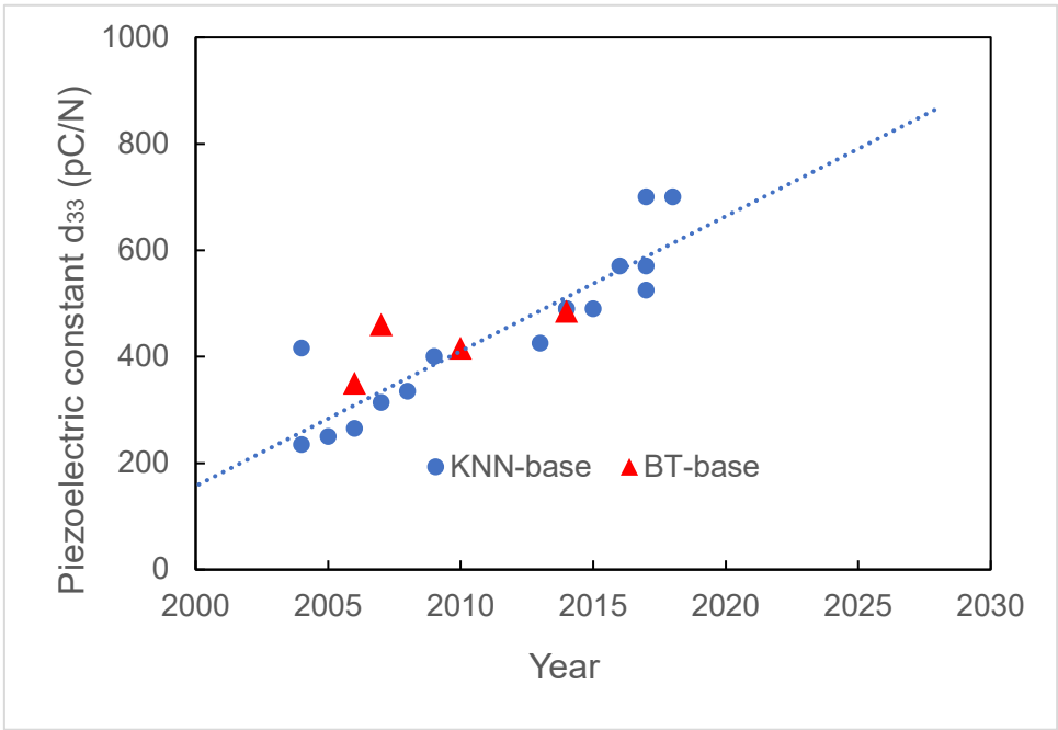
圧電アクチュエータへの応用が期待される非鉛圧電材料の圧電定数 d_{33} の傾向
