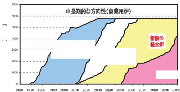
図1 原子力発電容量の見通し
