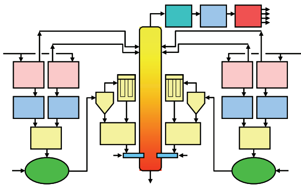
図2 炭化ガス化実験設備の概略系統
