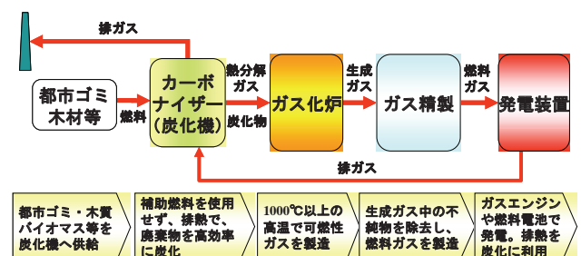
図1 炭化ガス化発電システム
