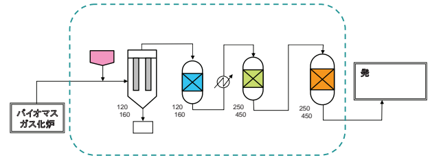
図4 乾式ガス精製設備の概略系統
